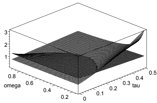
Fig. 4a,b: \Upsilon_a (dark), \frac{1}{\Upsilon_b} (light); \sigma = 0.075 , \rho = 0 , \mu = 0.075
