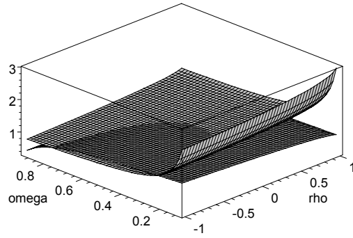
Fig. 2a,b: \Upsilon_a (dark), \frac{1}{\Upsilon_b} (light); \mu = 0.075 , \sigma = 0.075 , \tau = 0.25
