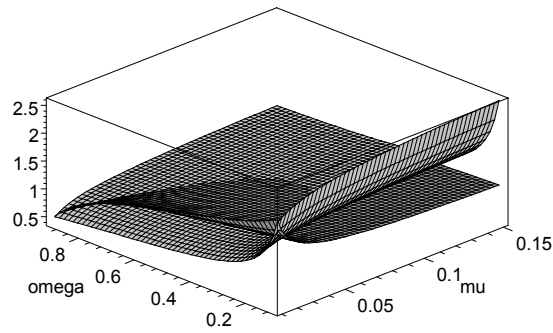
Fig. 3a,b: \Upsilon_a (dark), \frac{1}{\Upsilon_b} (light); \sigma = 0.075 , \rho = 0 , \tau = 0.25
