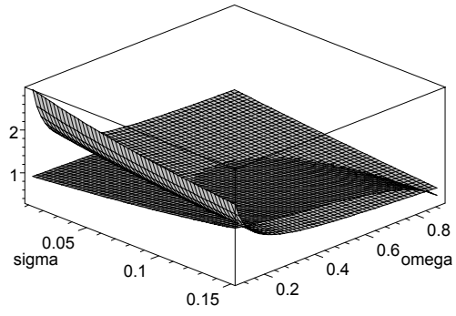
Fig. 1a,b: \Upsilon_a (dark), \frac{1}{\Upsilon_b} (light); \mu = 0.075 , \rho = 0 , \tau = 0.25
