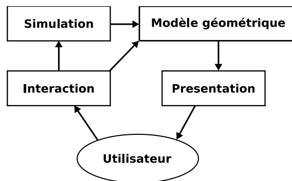
FIG. 2.2 – La décomposition proposée par le Decoupled Simulation Model
