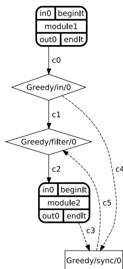
FIG. 12.5 – Schéma greedy entre 2 modules
