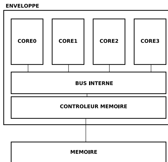
FIG. 3.2 – Processeur doté de 4 coeurs et d'un contrôleur mémoire intégré
