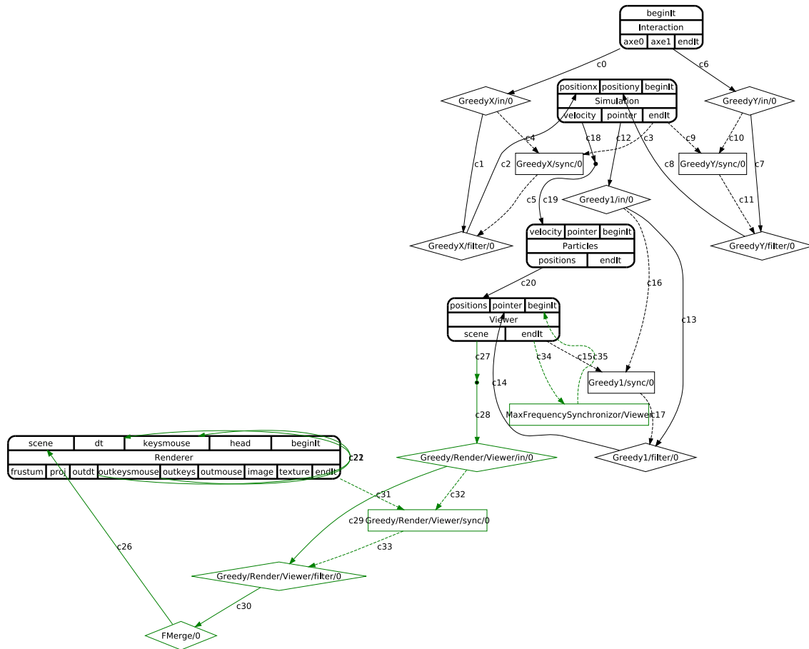
FIG. 12.2 – Organisation de l'application FluidParticle
