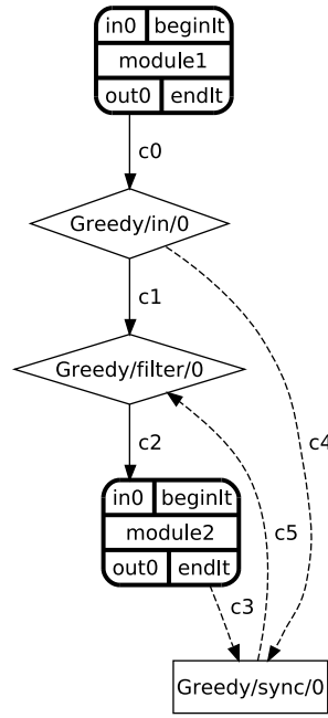
FIG. 7.2 – Schéma de connexion greedy entre deux modules
