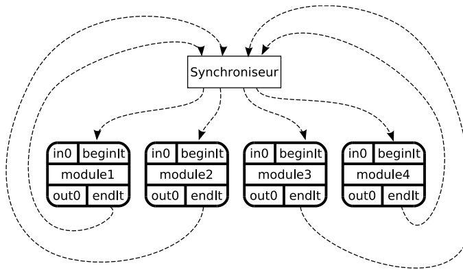
FIG. 7.7 – Synchronisation de plusieurs modules
