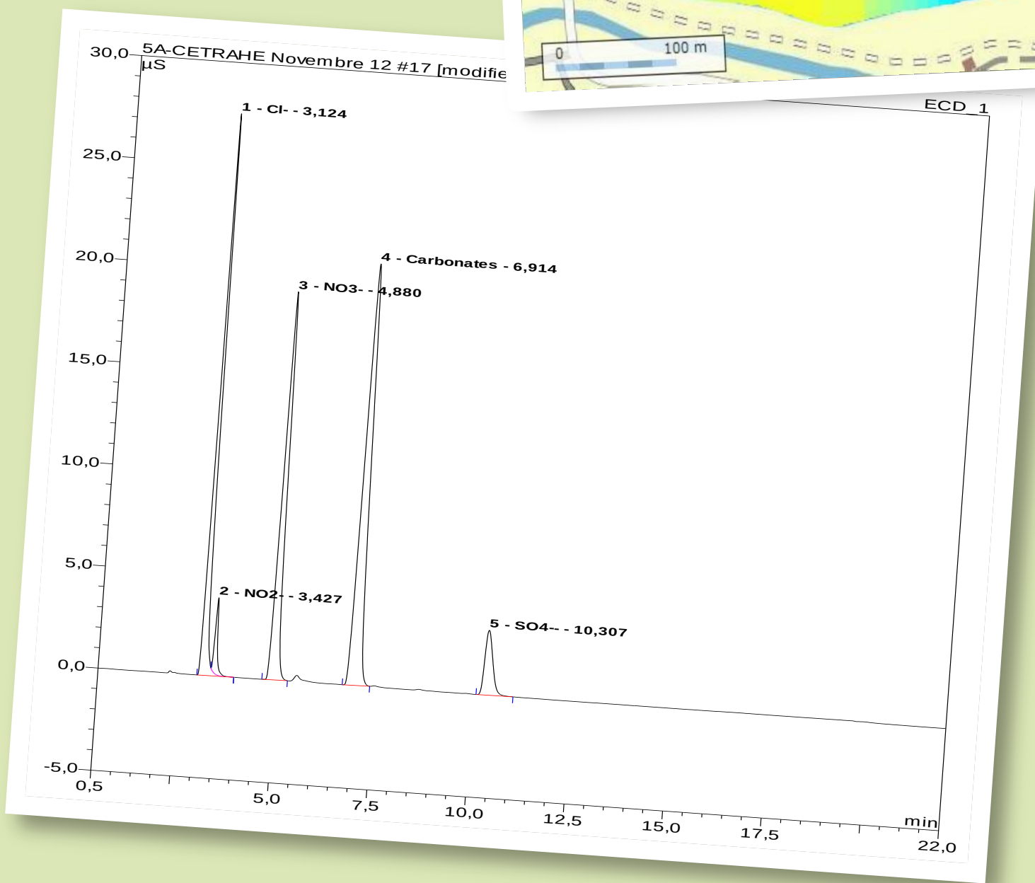
Chromatogramme de la composition chimique de l'eau
